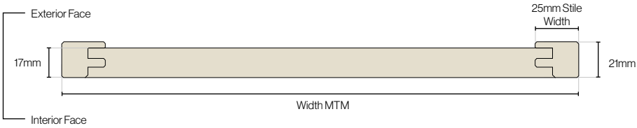
Brooklyn Door Cross Section
